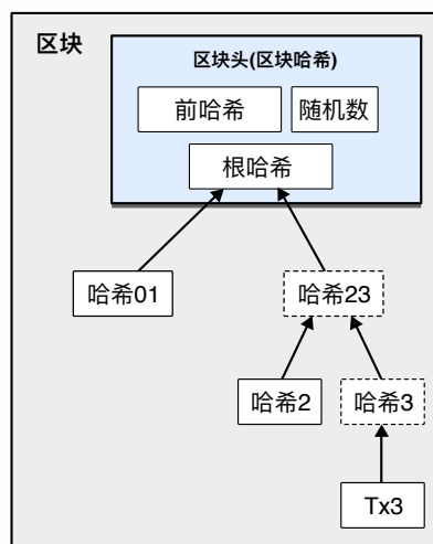
从区块里剪除 Tx0-2 之后
