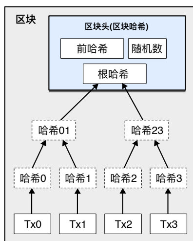
交易的哈希以 Merkle 树方式组织
